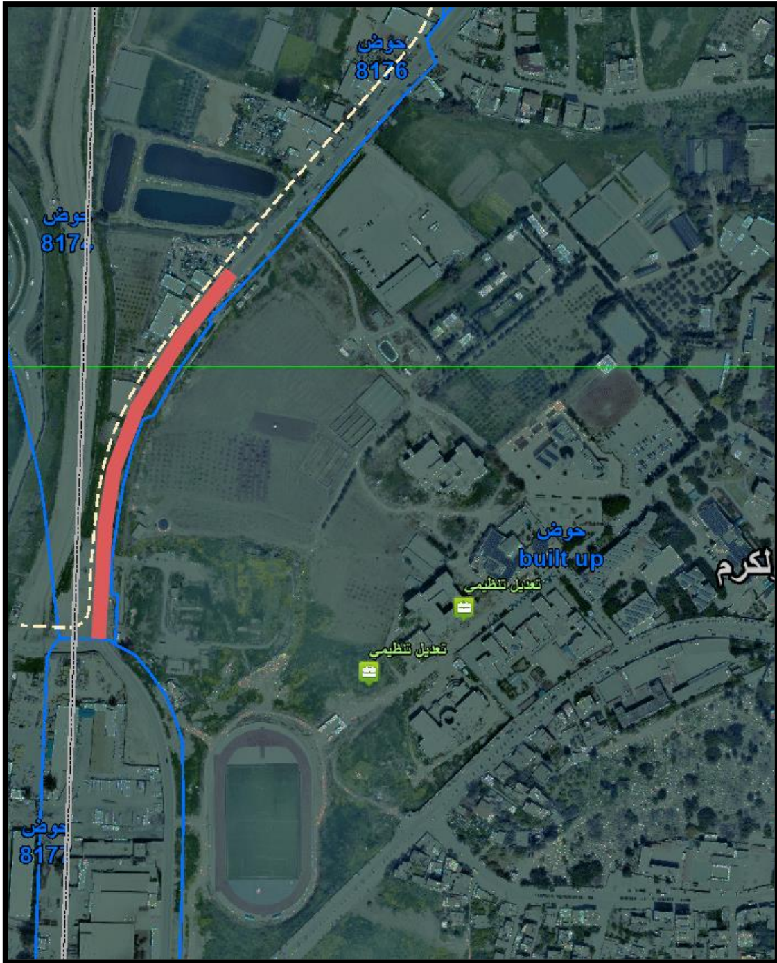
خط الكهرباء من بوابة نتانيا حتى غرف الكهرباء في ارض جامعة خضوري
